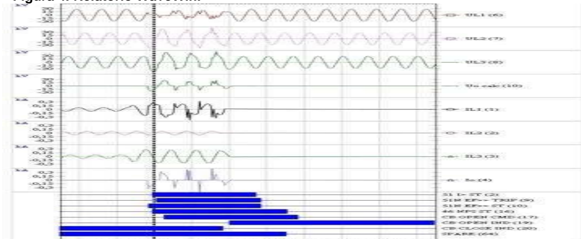
Figura 4. Relatório WaveWin.
