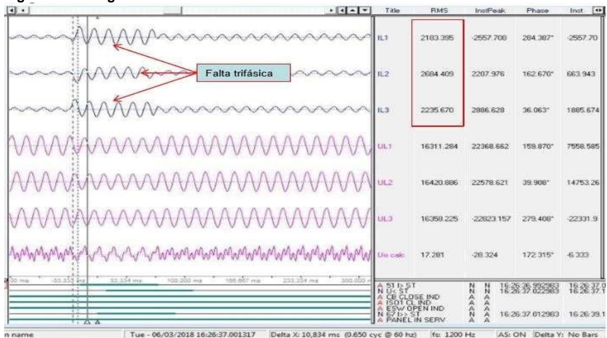
Figura 6. Oscilografia.
