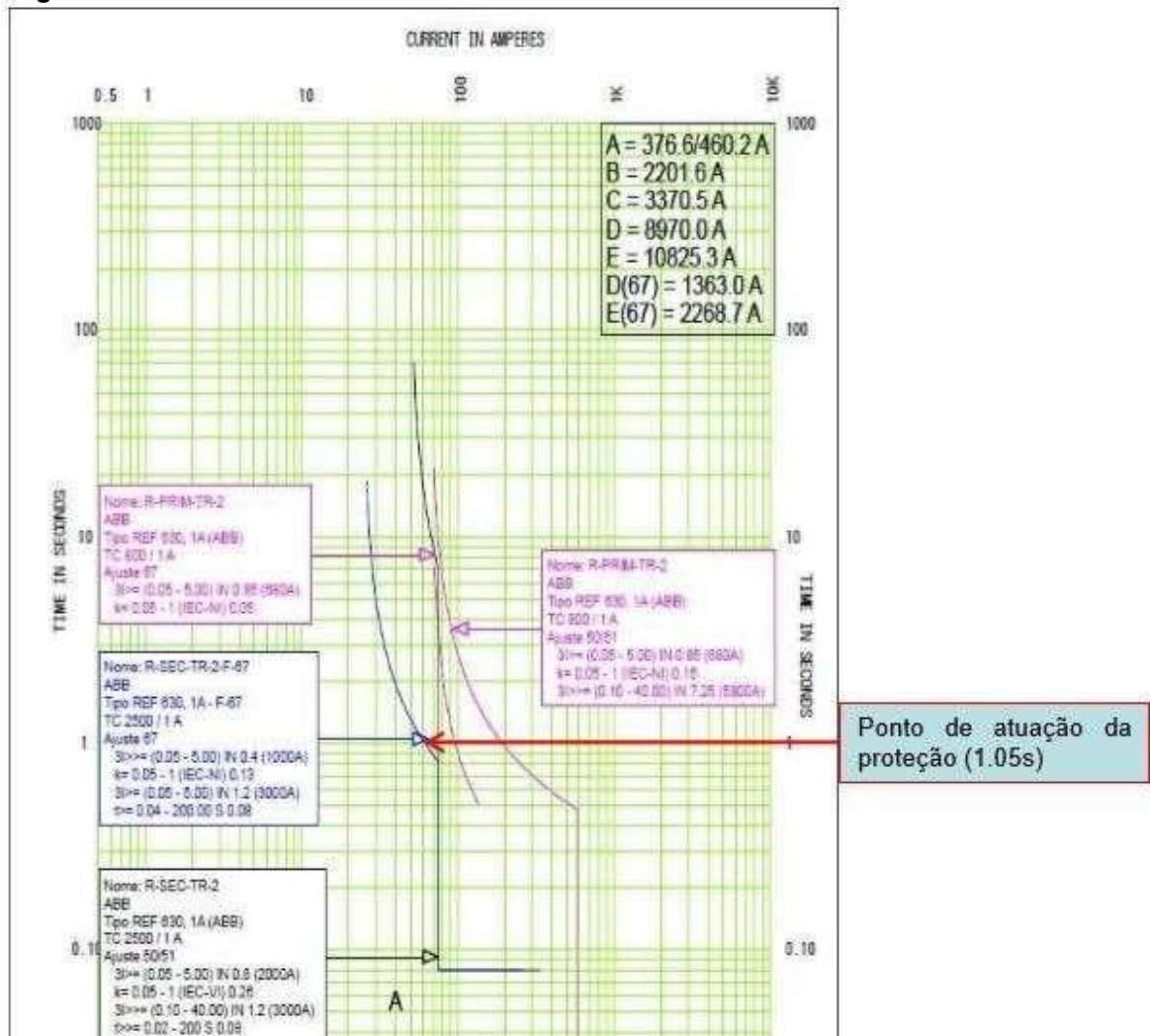
Figura 8. Curva IEC normal inversa.
